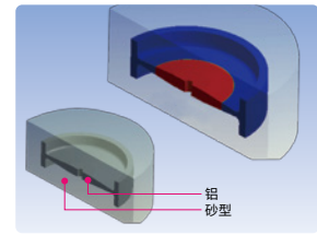
飞轮的铸造 (液体到固体的过渡阶段)
