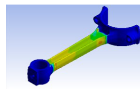
简谐应力载荷 Gerber 的平均应力修正结果
