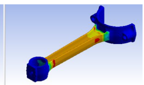
简谐应力载荷 Goodman 的平均应力修正结果
