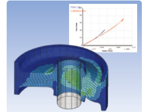
使用粘弹性-超弹性材料的橡胶衬套的应力分布
