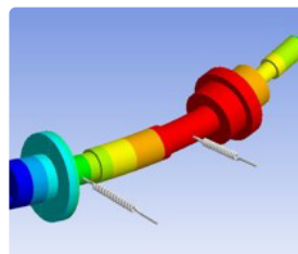
微型燃气轮机中的转子动力学
