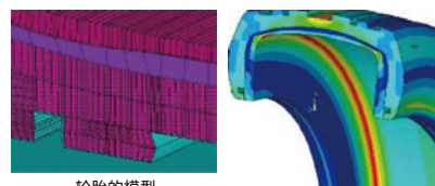
轮胎的模型 (在网格中输入加固材料的信息)
