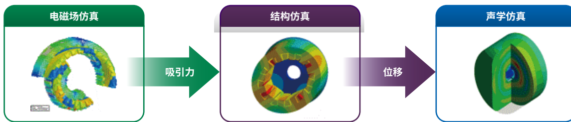
电机的电磁场 - 结构 - 声学耦合仿真
