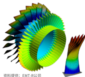
飞机风机的空气动力学弹性仿真
