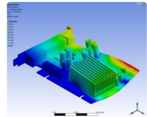
电路板的随机振动
