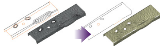
虚拟拓扑技术形状简化(去除微小的特征)
