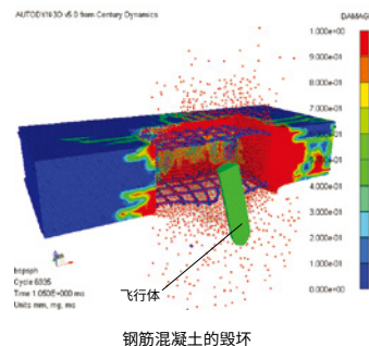
钢筋混凝土的破坏
