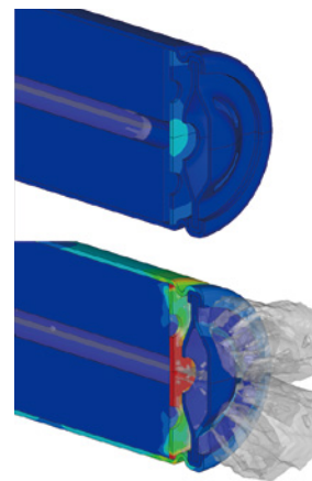
电池内部的流固耦合分析
