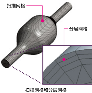
扫描网格和分层网格
