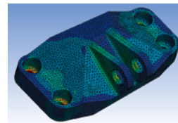
初始形状的应力分布
