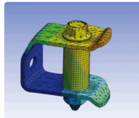
拧紧力引起的螺栓的应力 (螺栓预紧功能)
