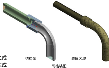
网格装配
