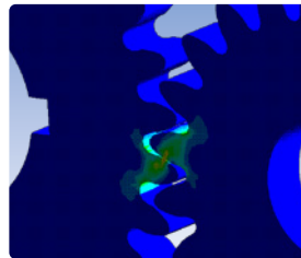
齿轮啮合 (接触)
