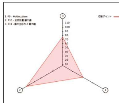
蜘蛛图
