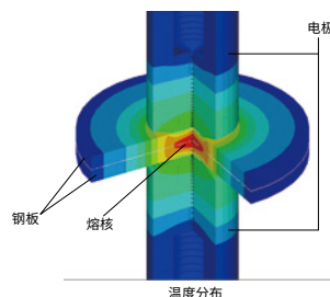
温度分布
