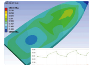
电焊斗的瞬态热仿真
