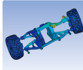
行驶部件的应力仿真
