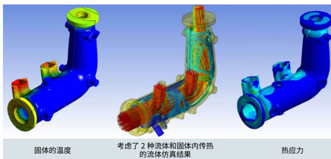
对燃气发动机排气管的集流管在 Ansys Workbench 环境中进行的 FSI 热应力仿真
