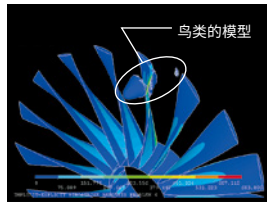
碰撞仿真结果（鸟类作为椭圆形建立模型）
