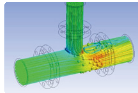
接头附近的热流体仿真
