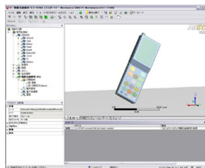
用 Ansys LS-DYNA 进行的手机跌落分析 (分析所需的设置均可以在 Ansys Workbench 环境中进行)
